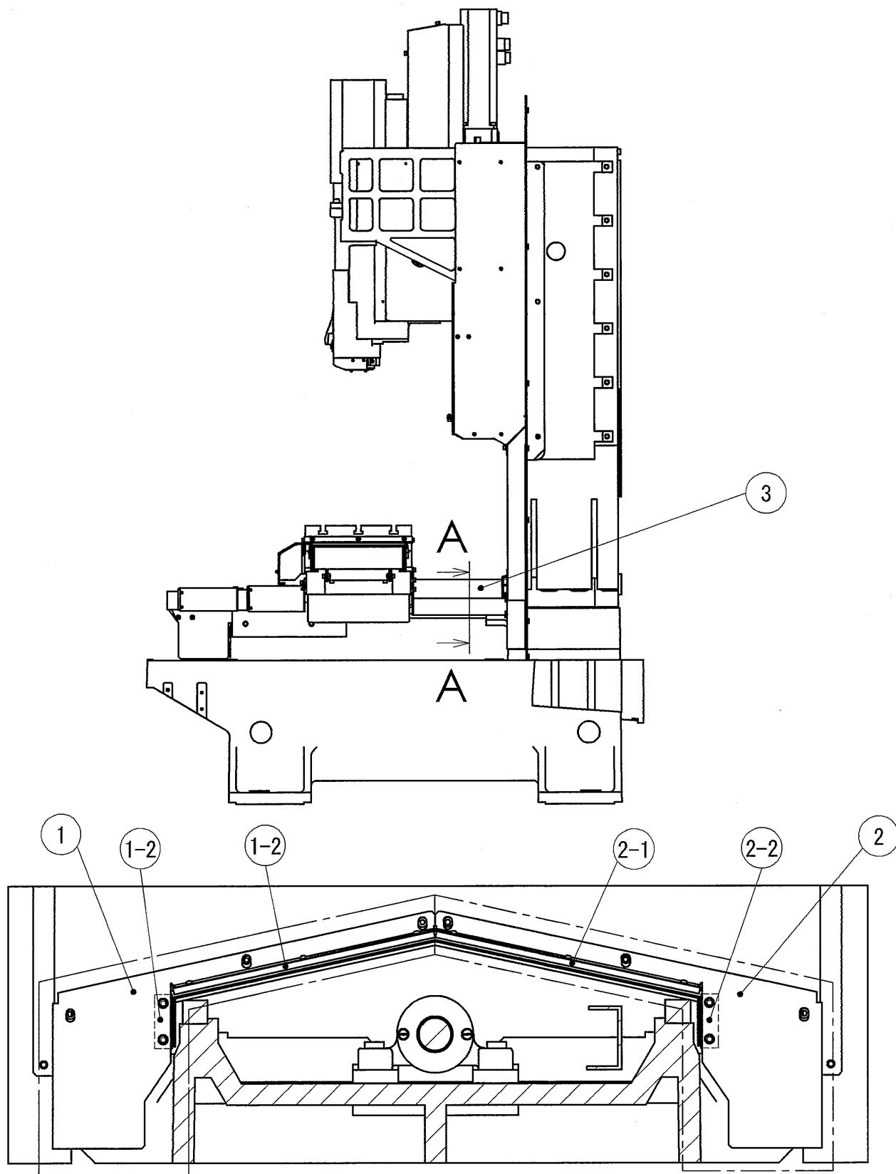
A-A (1 : 5)
